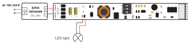
Рис. 1. Схема подключения диммера SMART-CC-201-72-DIM-IN для управления DIM-нагрузкой
